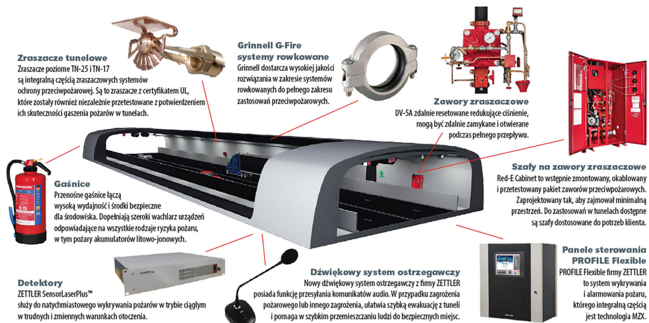
Fot. 2. Elementy składowe Kompleksowego Systemu Zabezpieczenia Tuneli
